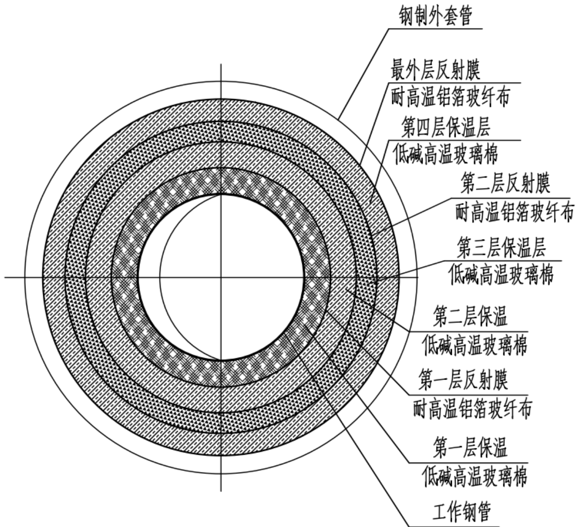
钢套钢直埋管保温结构大样图
